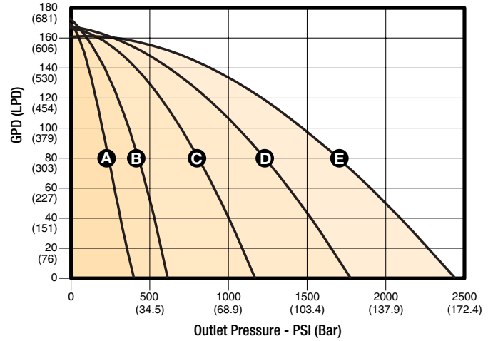
1/2" Plunger (PCI-250-50)
