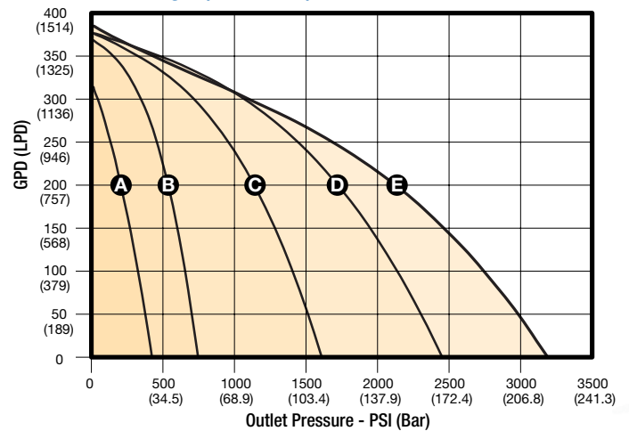
3/4" Plunger (PCI-450-75)
