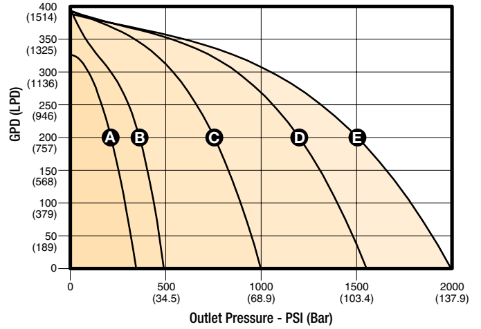
3/4" Plunger (PCI-450-75)
